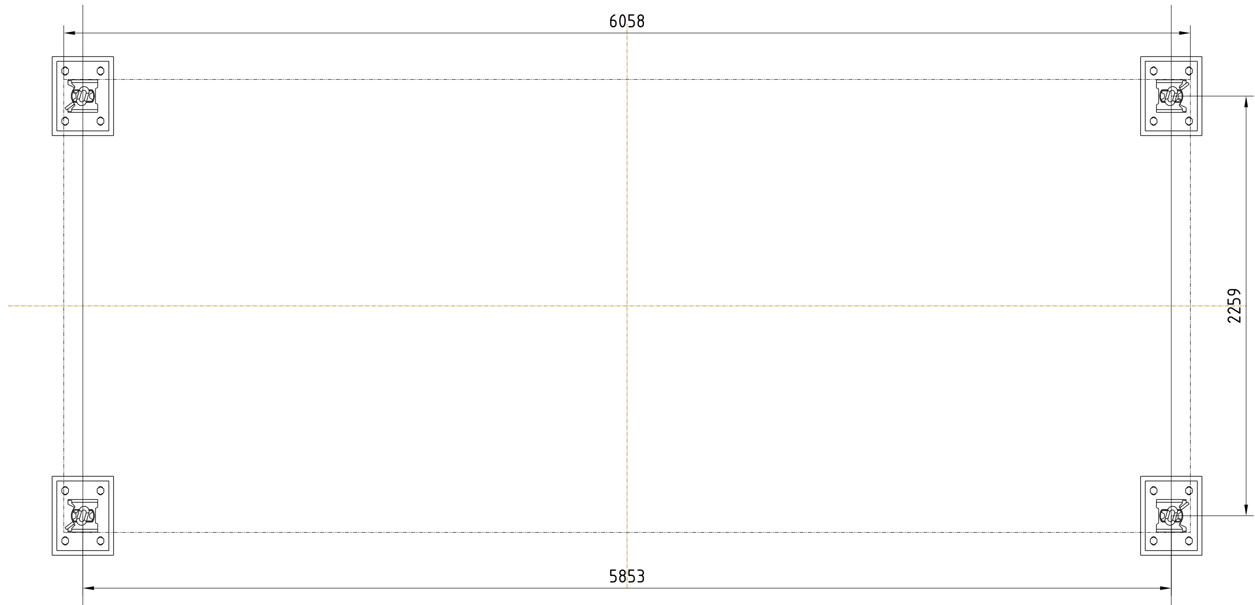
Опоры под модулем 20’ НС, М 1 : 20 (контур модуля – тонкой штрихпунктирной)
