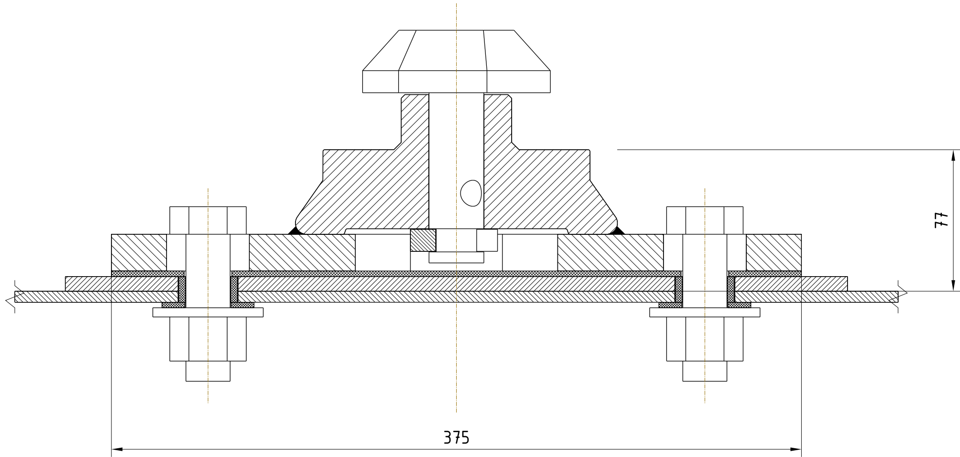
Разрез по оси опоры и по болтам, М 1 : 2
